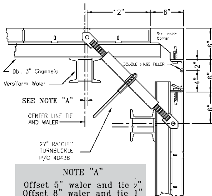
Double Hinged Filler (in pour position)
